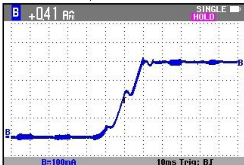
Рис. 9. Осциллограмма режима пуска при входном напряжении 220В, выходном напряжении 122В, выходной ток 400 мА
