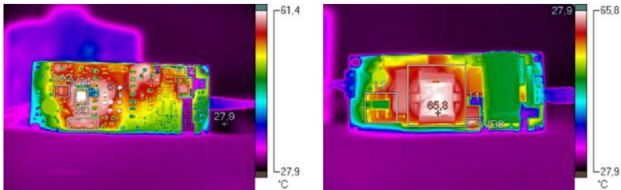
Рис. 19. Термограмма источника тока при входном напряжении 265 В, выходном напряжении 125 В, выходной ток 400мА
