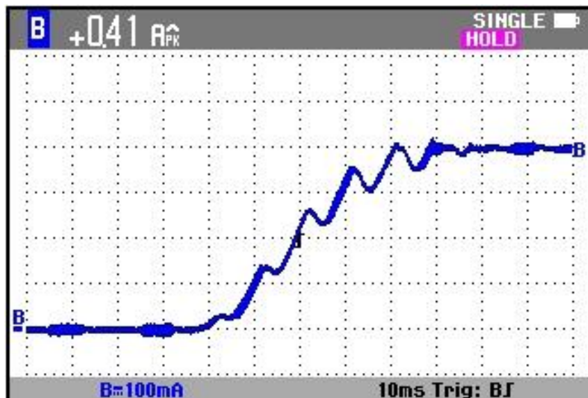
Рис. 8. Осциллограмма режима пуска при входном напряжении 160В, выходном напряжении 122В, выходной ток 400 мА
