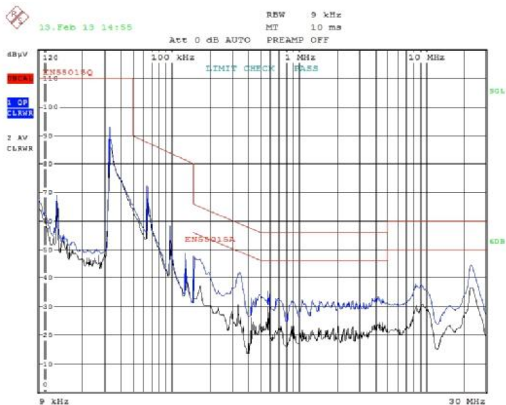
Рис. 16. Результаты тестирования источника тока на электромагнитную совместимость при выходном напряжении 65В, выходном токе 400 мА
