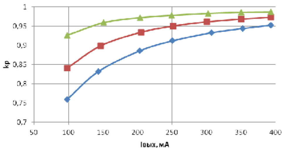
Рис. 5. Зависимость коэффициента мощности от выходного тока
